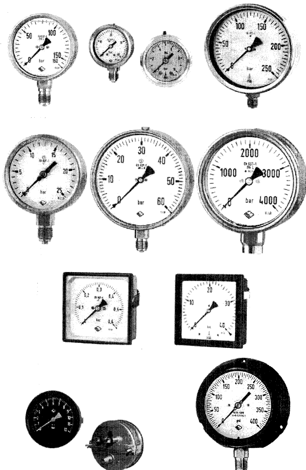
Slika 1. Fotografije manometara obuhvaćenih rješenjem
