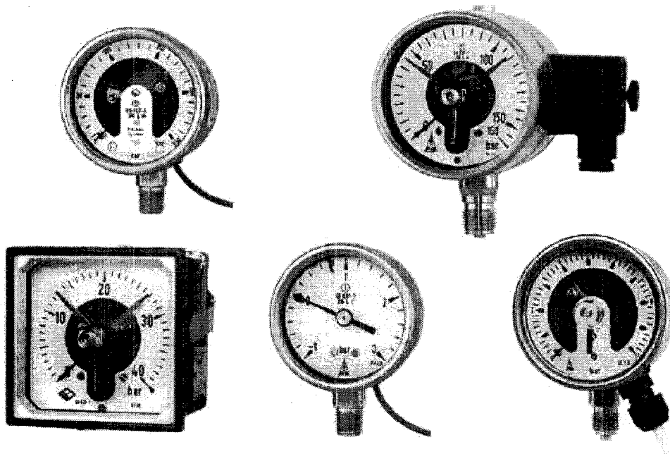
Slika 2. Manometri s električnim kontaktima
